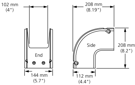
90° Down Elbow (FGS-MD9E-A)
