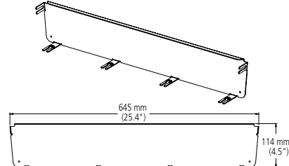
End Cap (FGS-HMEC-H)
