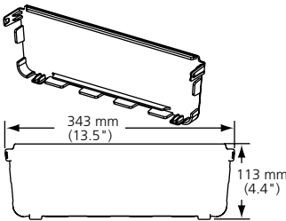
End Cap (FGS-HMEC-F)
