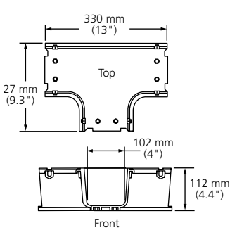
Horizontal T (FGS-MHRT-A)
